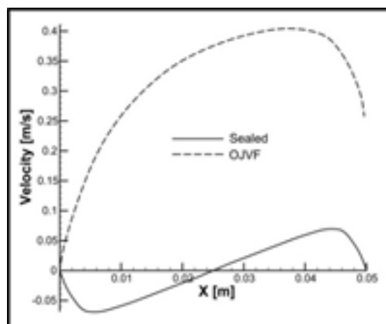
تصویر ۳ نیمرخ سرعت عمودی داخل حفره در میانه ارتفاع از دیوار داخلی به سمت قطعات نما (منبع: نگارندگان)
