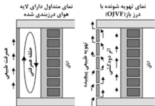
تصویر ۲: تفاوت رفتار هوای در نماهای باز و نمای بسته. ماخذ: [۱]
