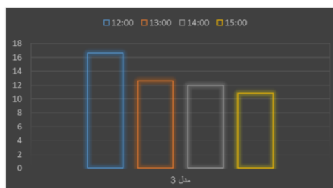
شکل ۱۶. مقادیر تغییر دمای سطح روسازی میدان در مدل ۳ برای ساعات میانی روز (از ۱۲ تا ۱۵ بعد از ظهر) در رسپتور ۱
