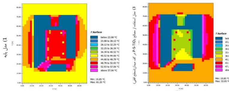
شکل ۱۵. نقشه توزیع میانگین دمای سطح روسازی میدان جلغا در مدل پایه و مدل ۳ (ساعت ۱۳ عصر)
