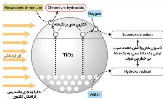
شکل ۲. واکنش‌های فوتوکاتالیستی روی سطح ماده TiO_2
