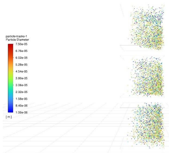
شکل ۱۲- کانتور قطر ذرات در داخل حفره‌های هر فرم (دید عریضی) (نویسنده‌گان)
