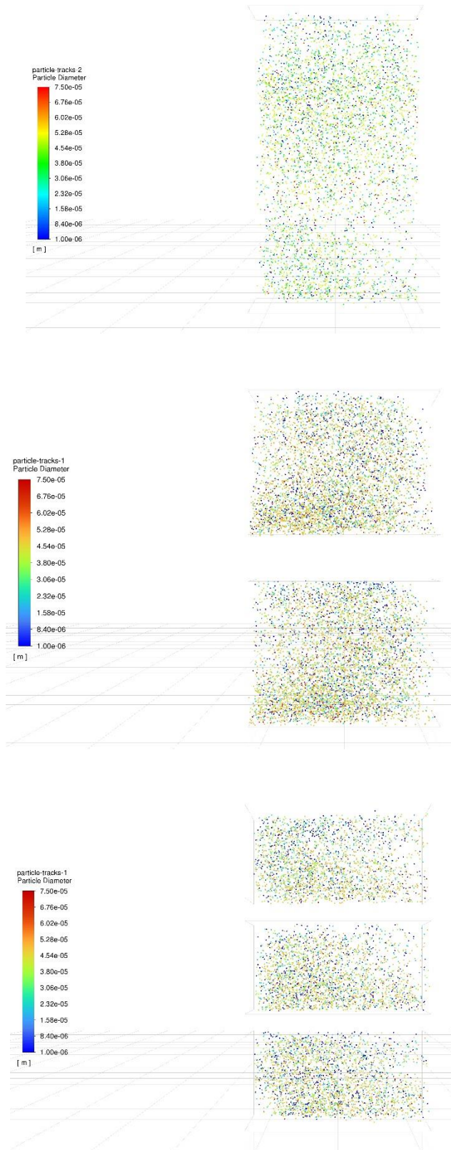
شکل ۱۱- کانتور قطر ذرات در داخل حفره‌های هر فرم (دید افقی) (نویسنده‌گان)
