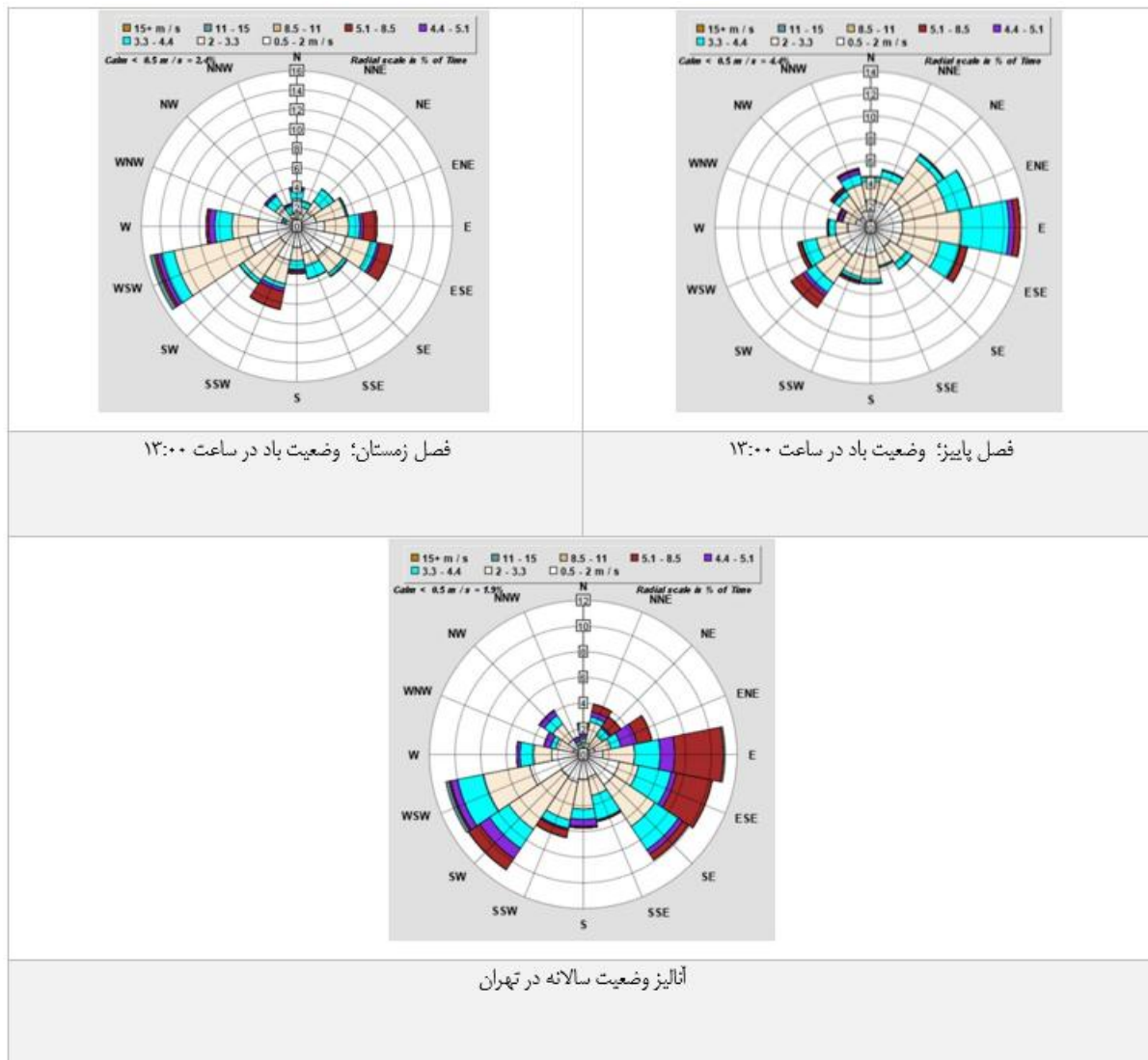
جدول ۳- بررسی وضعیت باد در تمام ماه‌های سال و به طور سالیانه براساس مدل‌سازی ساختمان ویلایی ساخته شده در تهران؛ مدل‌سازی در نرم افزار Revit و نتایج در سایت Green Building Studio؛ منبع نگارندگان
