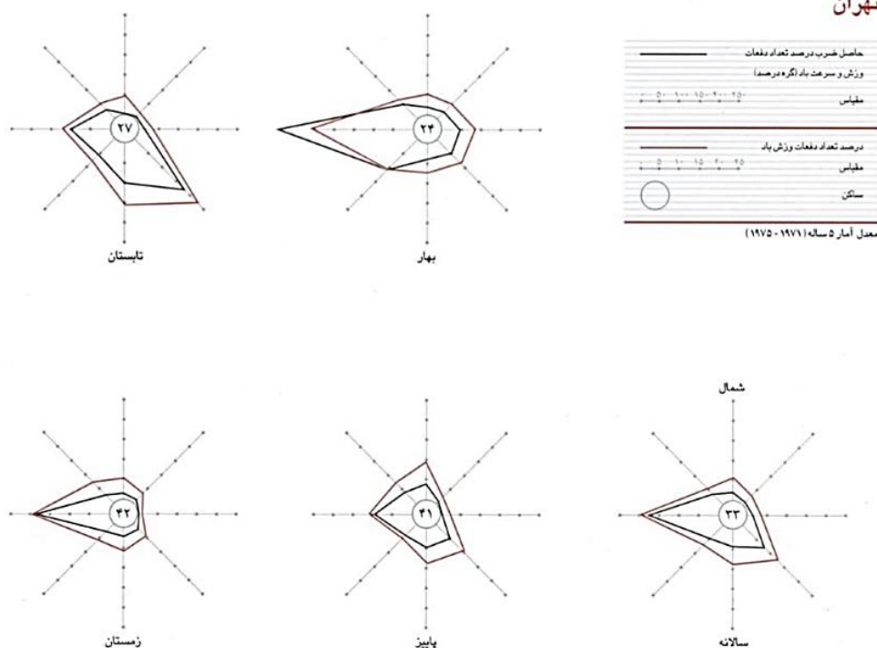
نمودار ۴- جهت و سرعت وزش باد در تهران؛ منبع کمسای
