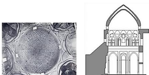
تصویر ۱۸: گنبد با باریکه طاق‌های باربر مقطع از گنبد مسجد جامع اردستان (Ashkan, 2009, 105) و نمای زیر گنبد مسجد جامع اردستان (معماریان، ۱۳۶۷، ۲۰۲).
