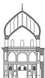
تصویر ۱۳: گنبد دو پوسته گسسته مسجد امام اصفهان مقطع گنبد (Ashkan, 2009, 109). و نمای داخلی گنبد مسجد امام اصفهان و نورگیرهایش (حاجی قاسمی، ۱۳۷۵، ۲۵).
