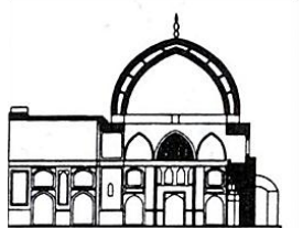
تصویر ۱۵: گنبد دو پوسته گسسته مسجد جامع یزد. مقطع گنبد (پیرنیا، ۲۳۴، ۱۳۸۶) و نمای خارجی گنبد مسجد جامع یزد (حاجی قاسمی، ۱۳۷۵، ۱۷۱).
