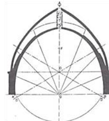
تصویر ۱۱: گنبد دو پوسته پیوسته بقعه سید رکن الدین یزد مقطع گنبد (پیرنیا، ۲۳۸، ۱۳۸۶). و نمای خارجی گنبد (www.mahoor.org)
