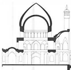
تصویر ۱۴: گنبد دو پوسته گسسته مسجد آقابزرگ کاشان. مقطع گنبد (حاجی قاسمی، ۱۳۷۵، ۱۵۷). و نمای خارجی گنبد آقابزرگ کاشان (حاجی قاسمی، ۱۳۷۵، ۱۵۳).
