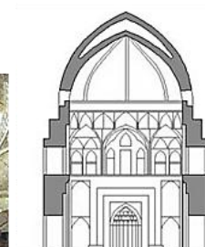
تصویر ۱۲: گنبد دو پوسته پیوسته مسجد برسیان اصفهان. مقطع گنبد (Ashkan, 2009, 105). و نمای زیر گنبد مسجد برسیان (www.shw.kousha.fotopages.com).
