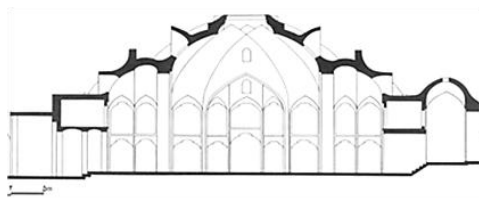
تصویر ۱۶: گنبد با باریکه طاق‌های باربر تیمچه ملک در بازار تبریز. (حاجی قاسمی، ۱۳۹۰، ۱۳۷۵). و نمای زیر گنبد تیمچه ملک. (حاجی قاسمی، ۱۳۷۵، ۱۳۷).
