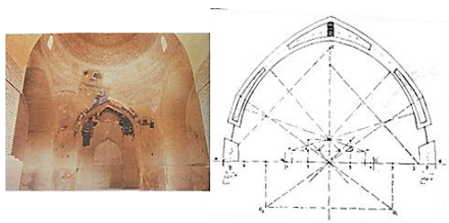
تصویر ۱۰: گنبد دو پوسته پیوسته مسجد کبود تبریز. مقطع گنبد و ایجاد نورگیر از میان بخش پیوسته آن (پیرنیا، ۶۶، ۱۳۷۰). و نمای زیر گنبد (حاجی قاسمی، ۱۳۷۵، ۶۱).
