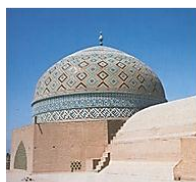
تصویر ۱۵: گنبد دو پوسته گسسته مسجد جامع یزد. مقطع گنبد (پیرنیا، ۲۳۴، ۱۳۸۶) و نمای خارجی گنبد مسجد جامع یزد (حاجی قاسمی، ۱۳۷۵، ۱۷۱).
