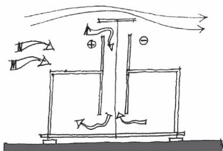
شکل ۹. در ساختار بادگیرها عضو ورودی و خروجی با هم در یک مجموعه تعبیه شده است. منبع: محمودی، ۱۳۸۸
