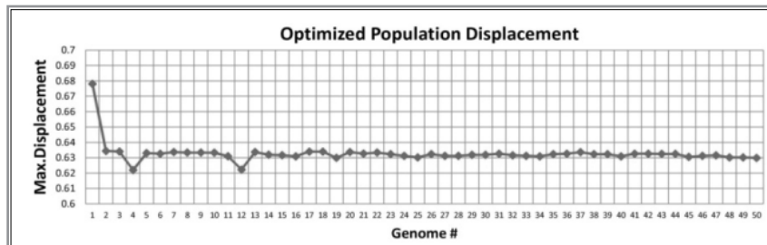
نمودار ۳-۳: روند تغییرات جابه‌جایی حداکثری اجزای تشکیل دهنده‌ی سازه در جمعیت بهینه
