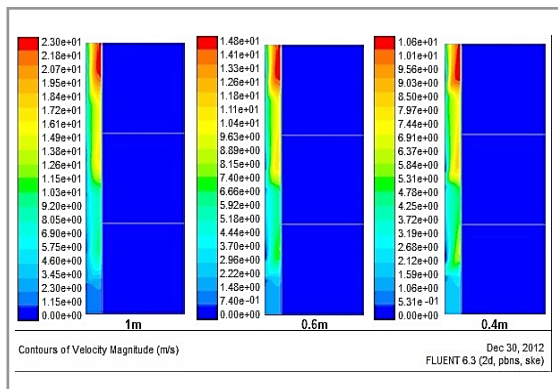
نمودار ۶: تغییرات سرعت هنگام شب در تابستان با سه دریچه باز روی نمای خارجی
