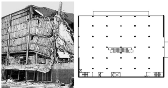
شکل (۱) تخریب ساختمان جی.سی.پنی در زلزله ۱۹۶۴ آلاسکا در اثر پیچش ناشی از چیدمان دیوارها [1]
