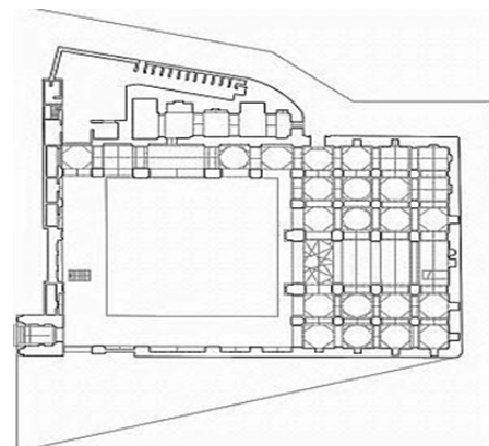
شکل ۱۴) پلان مسجد جامع دزفول (اداره میراث فرهنگی)
