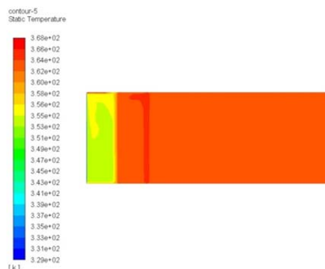
شکل ۴) کانتور دما در مقطع عرضی حالت دوم
