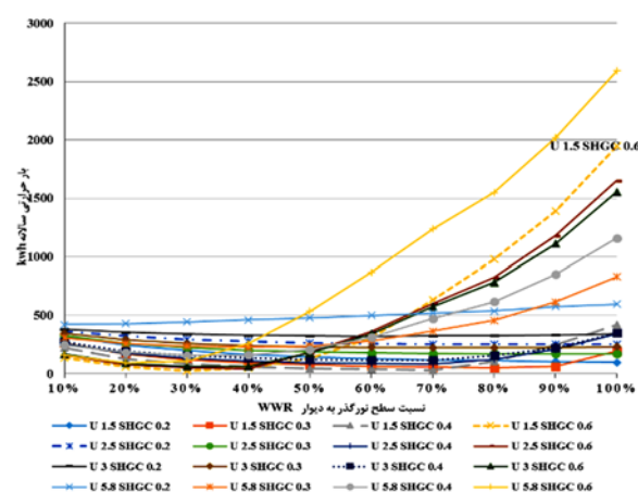
نمودار (۵) بار حرارتی و برودتی سالانه کلاس با پوسته خارجی دیوار سه‌بعدی (3DP) [26]
