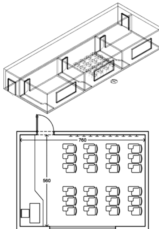
شکل ۱) ابعاد و موقعیت کلاس شبیه‌سازی شده در نرم‌افزار دیزاین‌بیلدر [26]
