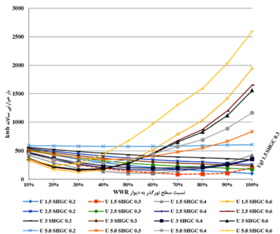
نمودار ۳) بار حرارتی و برودتی سالانه کلاس با پوسته خارجی دیوار بلوک سفالی (HCB) [26]
