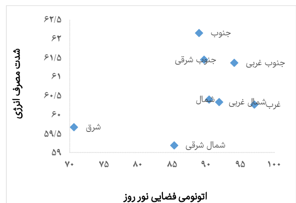
نمودار ۱) نمودار نسبت اتونومی نور فضایی به انرژی مصرفی در مدل‌های بهینه
