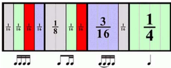
شکل ۵) نسبت‌های موزون ریاضی میان چهار نت موسیقی؛ برگرفته از سایت bewitched
