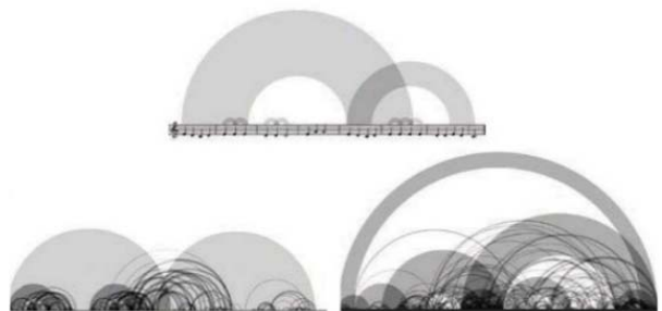
شکل ۳) دیگرام‌های قوسی ترسیم‌شده توسط مارتین واتنبرگ پژوهشگر معاصر، برای نمایش ساختار موسیقی در یک قطعه مدرن (تصویر چپ)، سونات سل ماژور باخ (تصویر میانی) و فورالیز بتهوون (تصویر راست)؛ برگرفته از سایت bewitched
