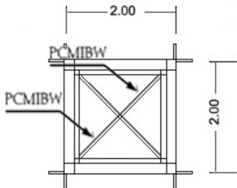
شکل ۸) برش عرضی بادگیر چهارطرفه مدل شده و استفاده از مواد تغییر فاز دهنده در تیغه‌های متقاطع در ساختار بادگیر
