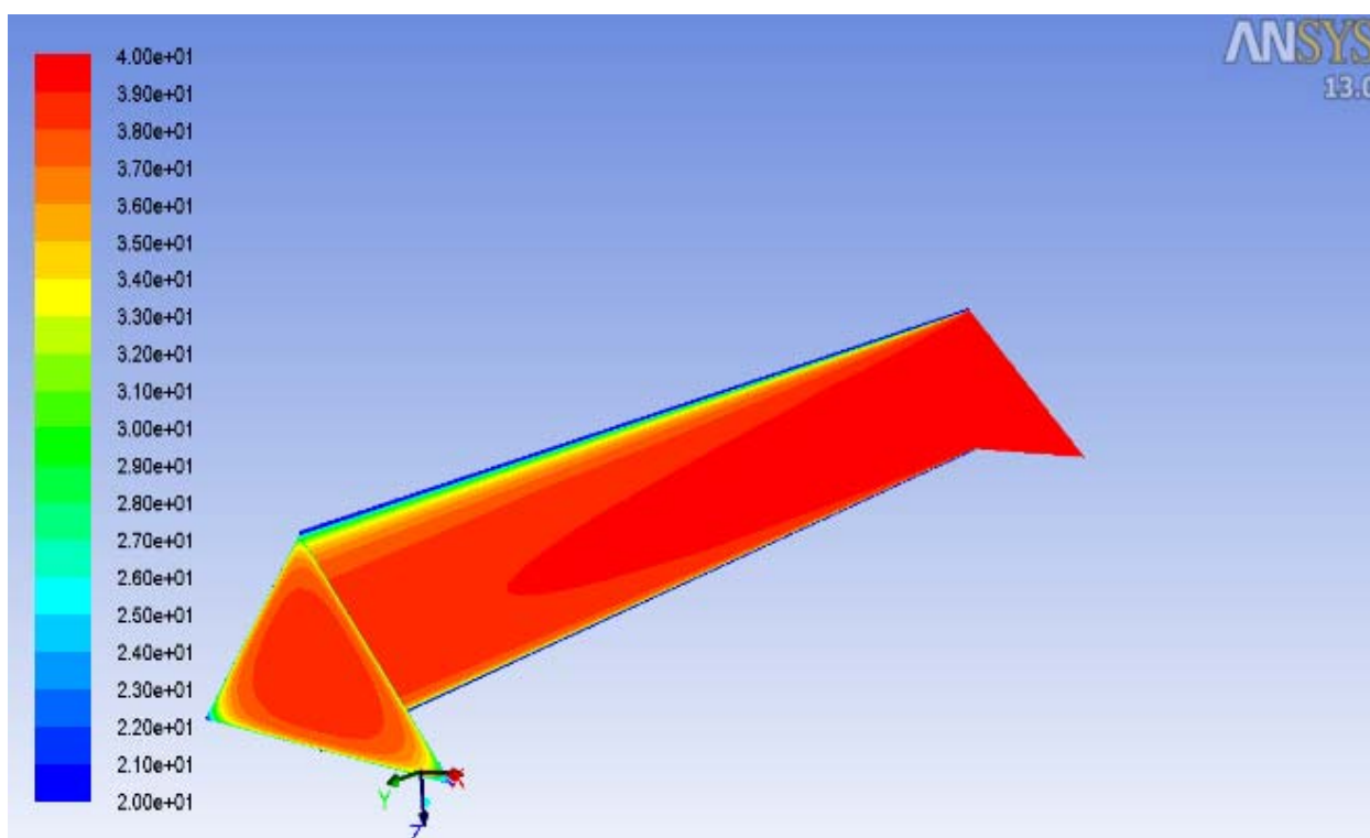
نمودار ۲) کانتورهای دمای کانال برای فایبرگلاس
