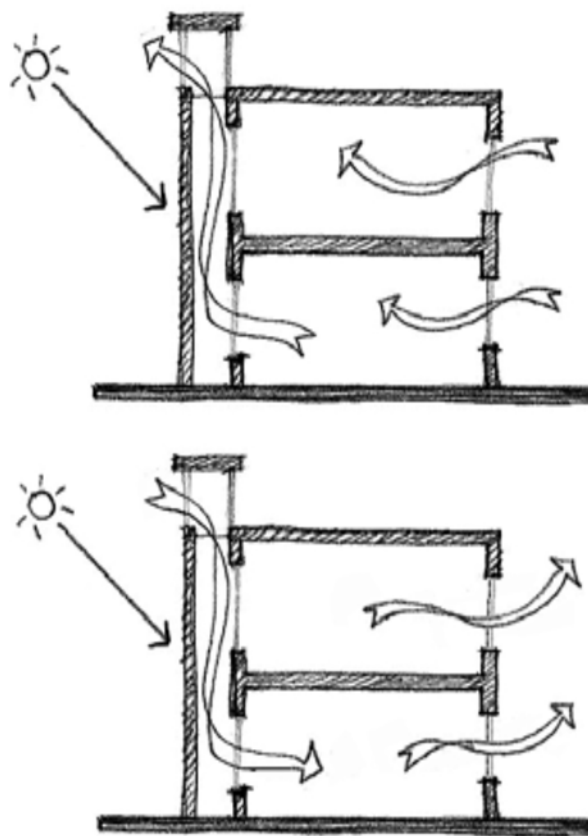
شکل ۲) نحوه تهویه در بادگیر [1]
