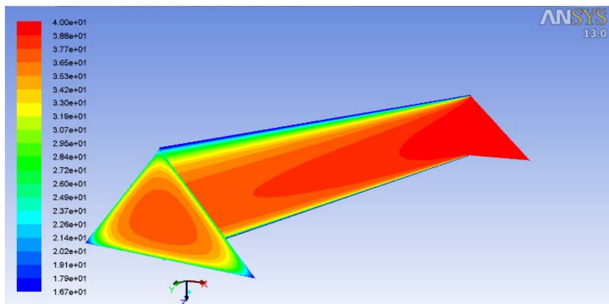
نمودار ۴) کانتورهای دمایی کانال برای PCM1
