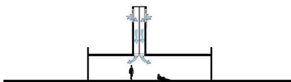
شکل ۷) برش ارتفاعی بادگیر مدل شده در فرآیند آزمایش
