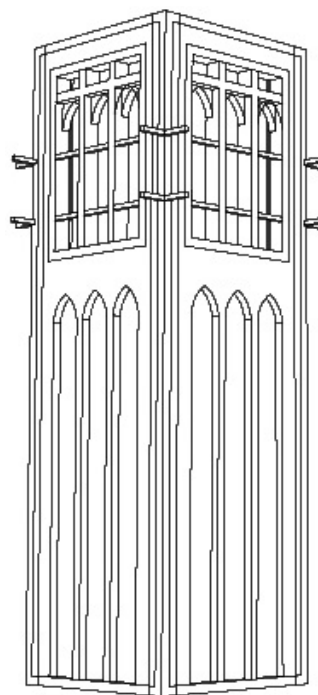
شکل ۵) ابعاد و نمونه بادگیر مدل شده در فرآیند آزمایش
