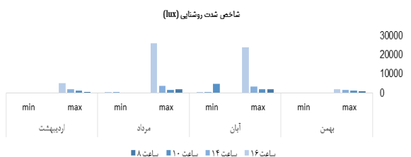
نمودار ۱۲) شاخص شدت روشنایی روز پانزدهم در کلاس ۲ دانشکده مکانیک و IT
