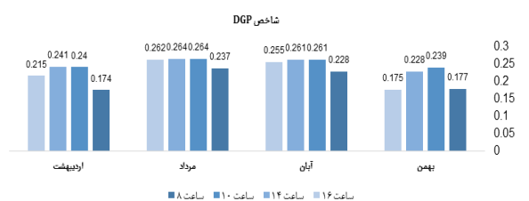
نمودار ۱۱) شاخص DGP روز پانزدهم در کلاس ۲ دانشکده مکانیک و IT
