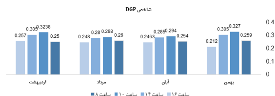
نمودار (۱) شاخص DGP روز پانزدهم در کلاس ۱ دانشکده فنی و مهندسی
