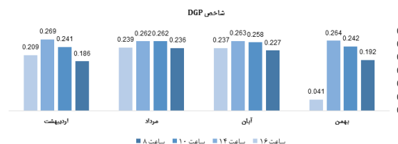
نمودار (۳) شاخص DGP روز پانزدهم در کلاس ۲ دانشکده فنی و مهندسی
