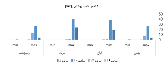
نمودار (۶) شاخص شدت روشنائی روز پانزدهم در کلاس ۳ دانشکده فنی و مهندسی
