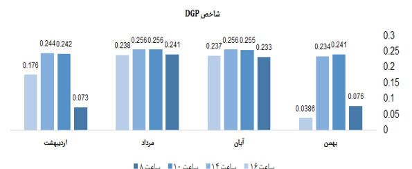
نمودار ۷) شاخص DGP روز پانزدهم در کلاس ۴ دانشکده فنی و مهندسی
