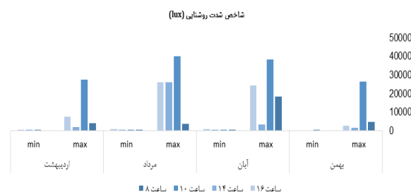
نمودار (۲) شاخص شدت روشنائی روز پانزدهم در کلاس ۱ دانشکده فنی و مهندسی
