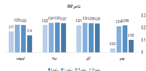
نمودار ۱۳) شاخص DGP روز پانزدهم در کلاس ۱ دانشکده علوم پایه
