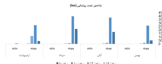
نمودار (۴) شاخص شدت روشنائی روز پانزدهم در کلاس ۲ دانشکده فنی و مهندسی
