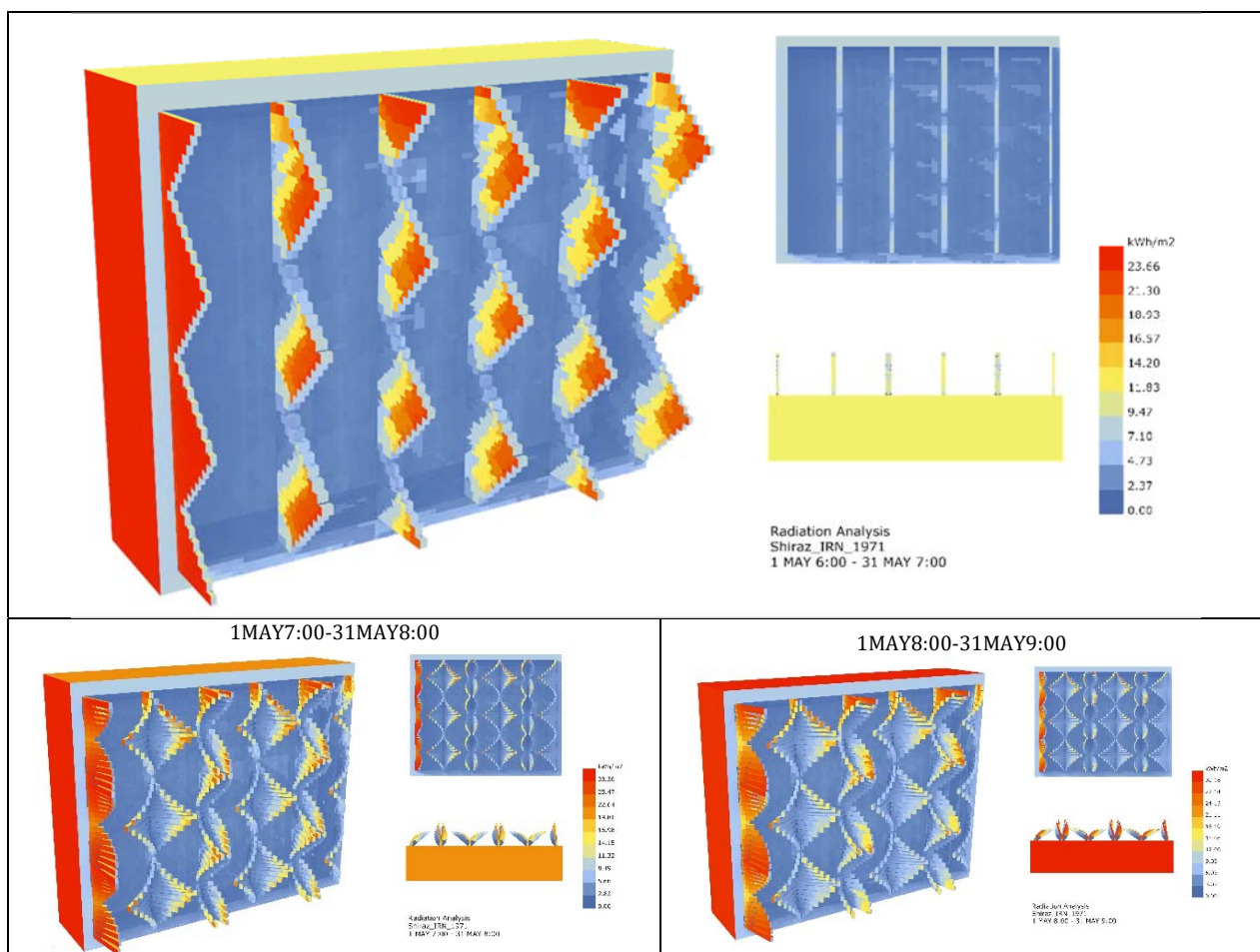
شکل ۵) تحلیل انرژی پوسته هوشمند الهام‌گرفته از الگوریتم حرکتی گیاه قهر و آشتی توسط افزونه گرس‌هپیر از ساعت ۶ تا ۱۹ در ماه مرداد و اقلیم شهر شیراز
