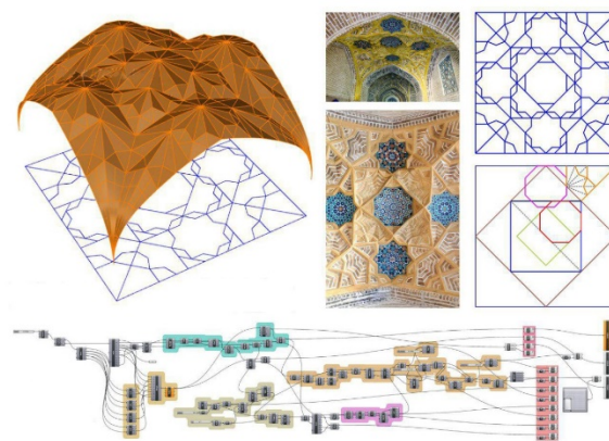
شکل ۱۰) کاسه‌سازی مدرسه کوکدش بخارا ازبکستان در نرم‌افزار راینو و گرس‌هاپر
