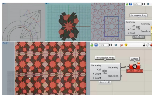
شکل ۹) طراحی پارامتریک یک نوع گره تند در نرم‌افزار راینو و گرس‌هاپر که قابلیت تغییر پارامترها و تکثیر در سطوح را دارد.
