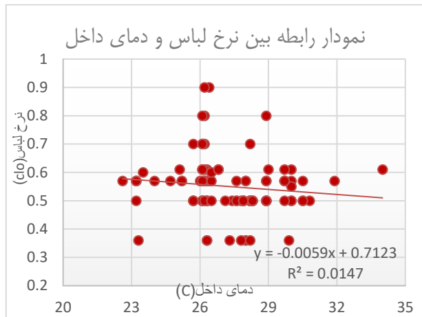
نمودار ۲- رابطه بین متغیر لباس و دمای هوای داخل
