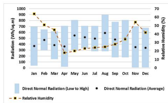
شکل ۴- میانگین وضعیت آب و هوای شیراز ۱۹۵۱-۲۰۱۰ (سازمان هواشناسی کشور) [۲۳]
