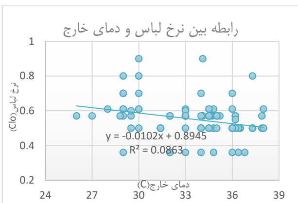
نمودار ۳- رابطه بین لباس و دمای هوای خارج در آپارتمان‌های شیراز
