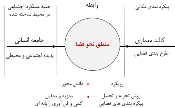
شکل ۱. تکنیک نحو فضا در ایجاد رابطه بین پیکره بندی مکانی و جنبه عملکرد اجتماعی
