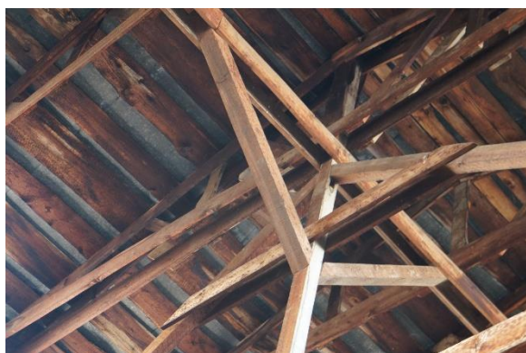
شکل ۱۹: جزئیات خرپای کارخانه نساجی شاهی
