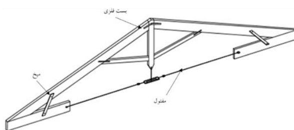
شکل ۲۷: جزئیات خرپای کارخانه شالیکوبی بابل
