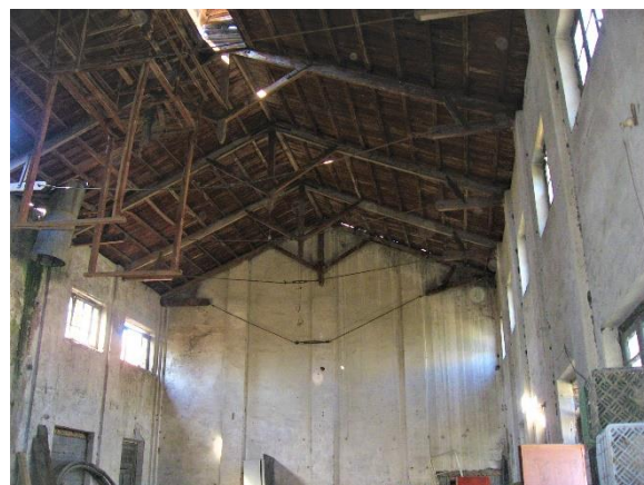
شکل ۲۶: خرپای کارخانه شالیکوبی بابل
