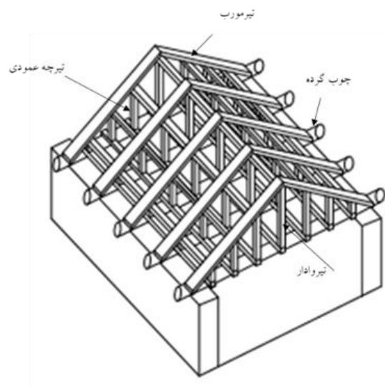
شکل ۱۴: جزئیات سازه شیبدار ساختمان فلاطوری لاهیجان
