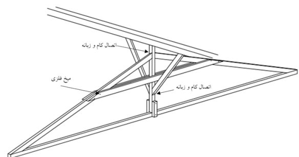
شکل ۲۷: جزئیات خرپای کارخانه پنبه بابلسر
