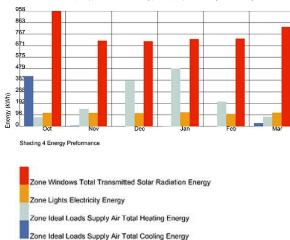
نمودار 6. نمودار تحلیل انرژی پسته با هندسه چهارم [نگارنده]
