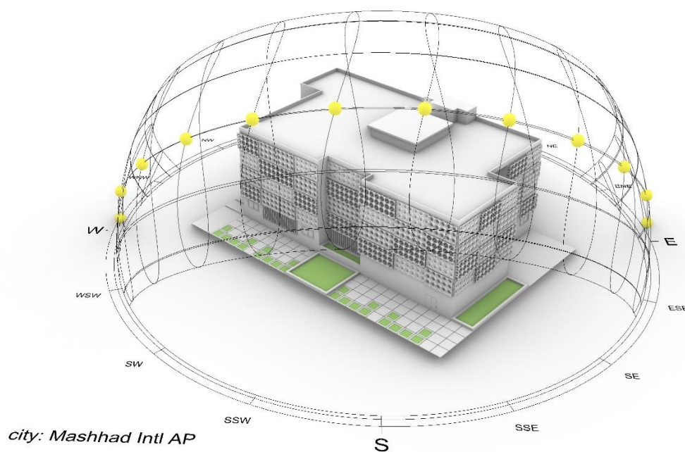
شکل 21. قرارگیری پوسته بر روی پروژه [نگارنده]
