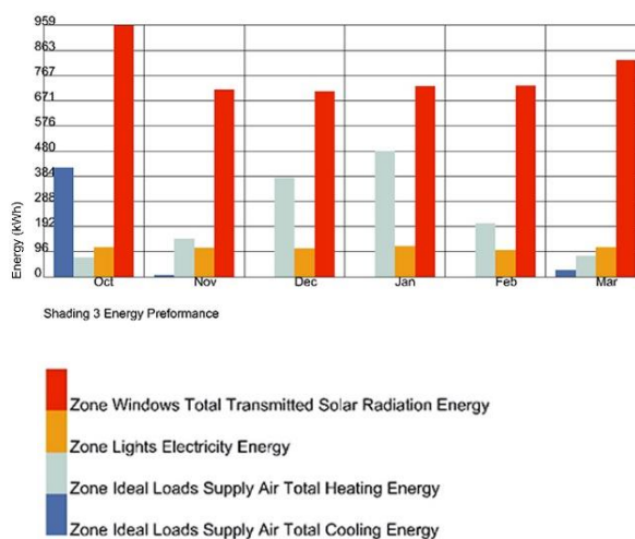
نمودار 5. نمودار تحلیل انرژی پوسته با هندسه سوم [نگارنده]
