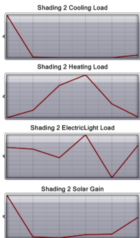
شکل 11. گراف آنالیز انرژی پوسته با هندسه دوم [نگارنده]
