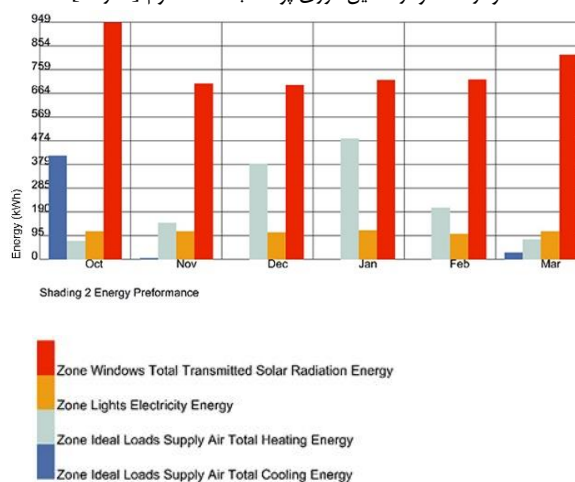
نمودار 4. نمودار تحلیل انرژی پوسته با هندسه دوم [نگارنده]
