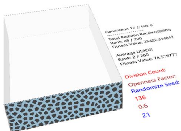
شکل ۲۰. طرح انتخابی برای پوسته غربی.
