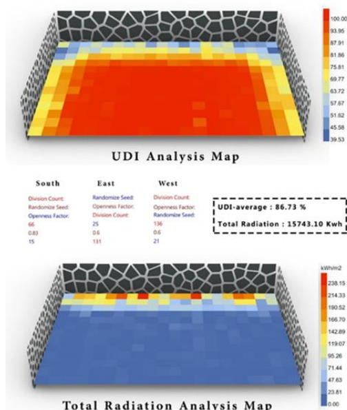
شکل ۲۳. نمودار آنالیز مدل سازی با طراحی پوسته ورونی.
