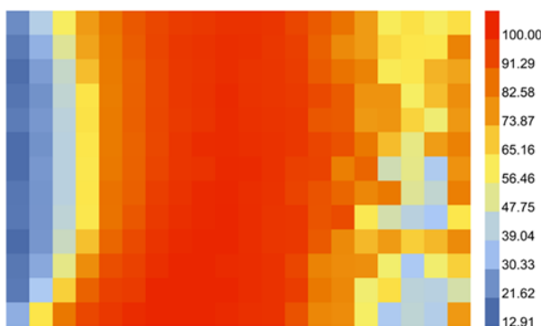
شکل ۸. آنالیز روشنایی مفید نور روز برای جبهه غربی.
