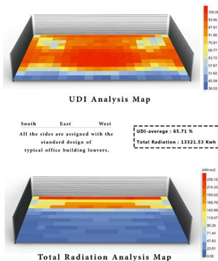
شکل ۲۲. نمودار آنالیز مدل‌سازی با به‌کارگیری لوور های افقی.
