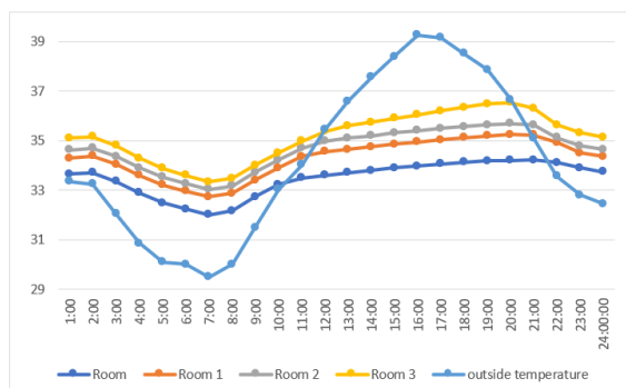
نمودار ۱ ( نمودار سمت راست): مقایسه تغییرات دما در سقف طبقات، منبع: نگارندگان
