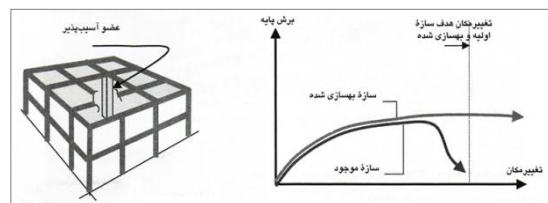
نگاره‌ی ۳. اصلاح موضعی اعضای سازه (مأخذ: محبی‌مقدم، ۳۴: ۱۳۸۷).
