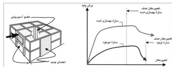
نگاره‌ی ۴. اصلاح کلی سیستم سازه‌ای (مأخذ: محبی‌مقدم، ۳۳: ۱۳۸۷).
