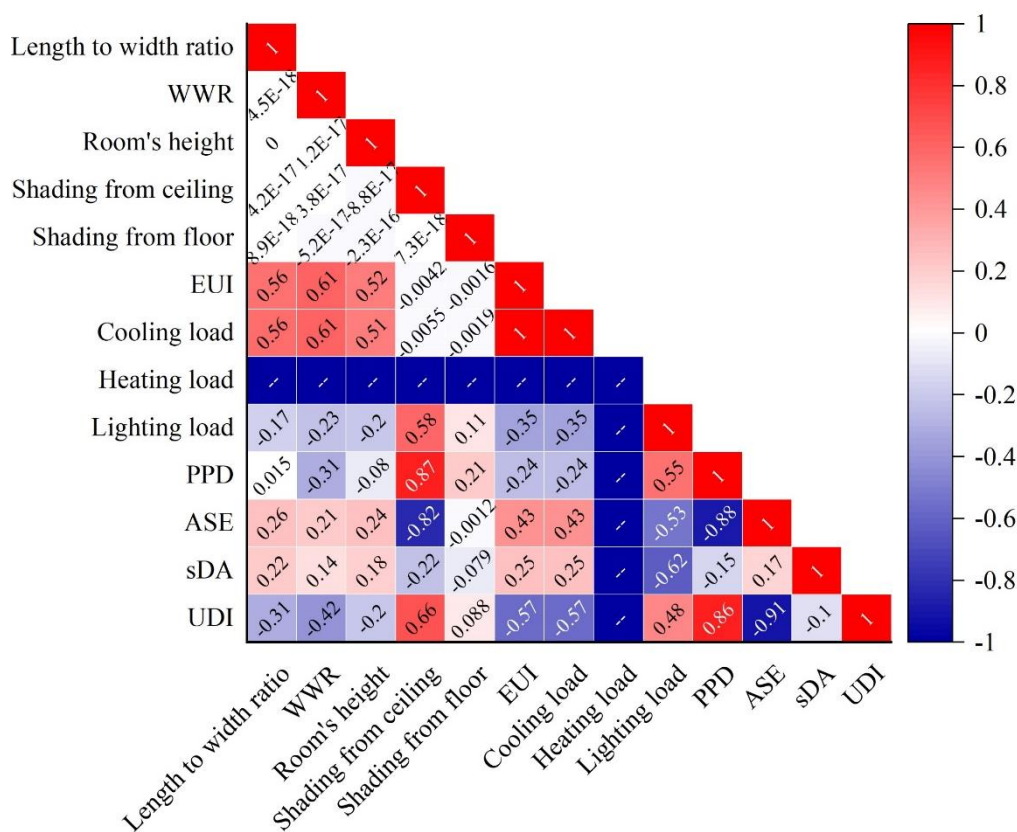
شکل ۹. آنالیز حساسیت
